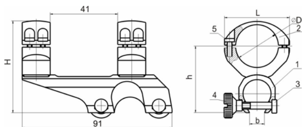
1. Основание 2. Охват 3. Винт стяжной 4. Гайка 5. Винт крепежный
